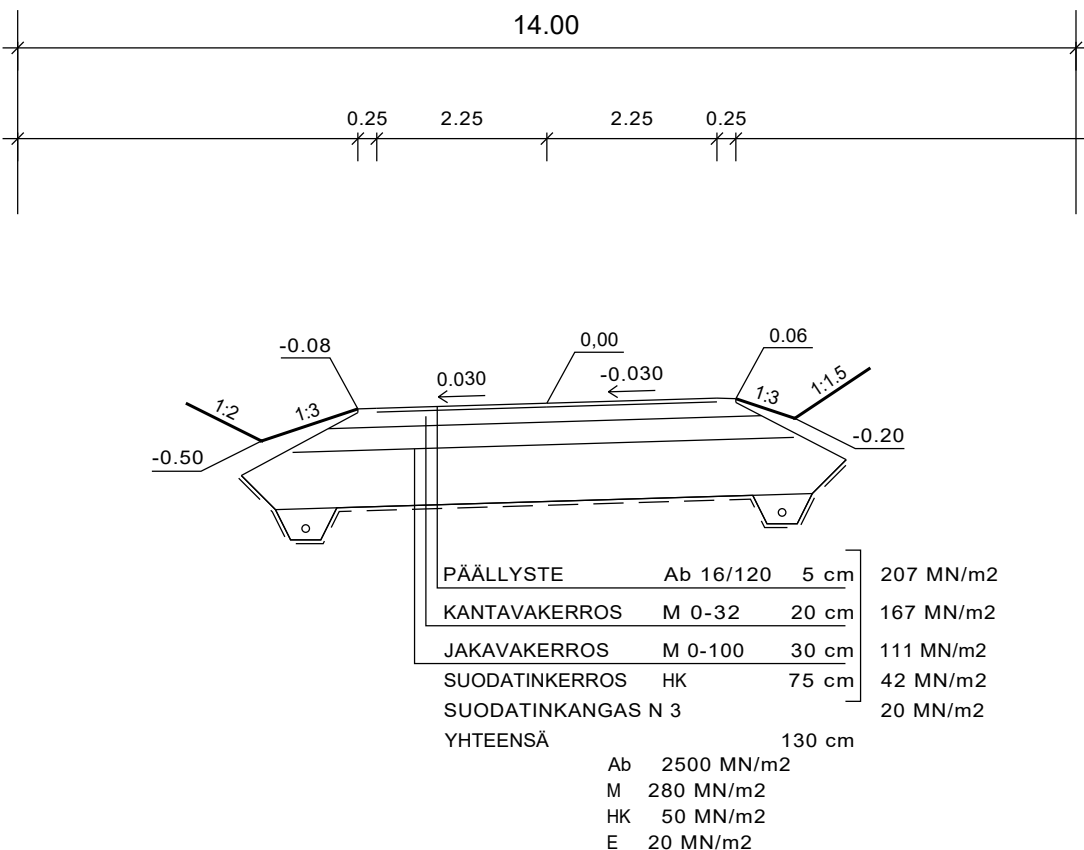
TYYPPIPOIKKILEIKKAUS PAALULTA 120 1:100
