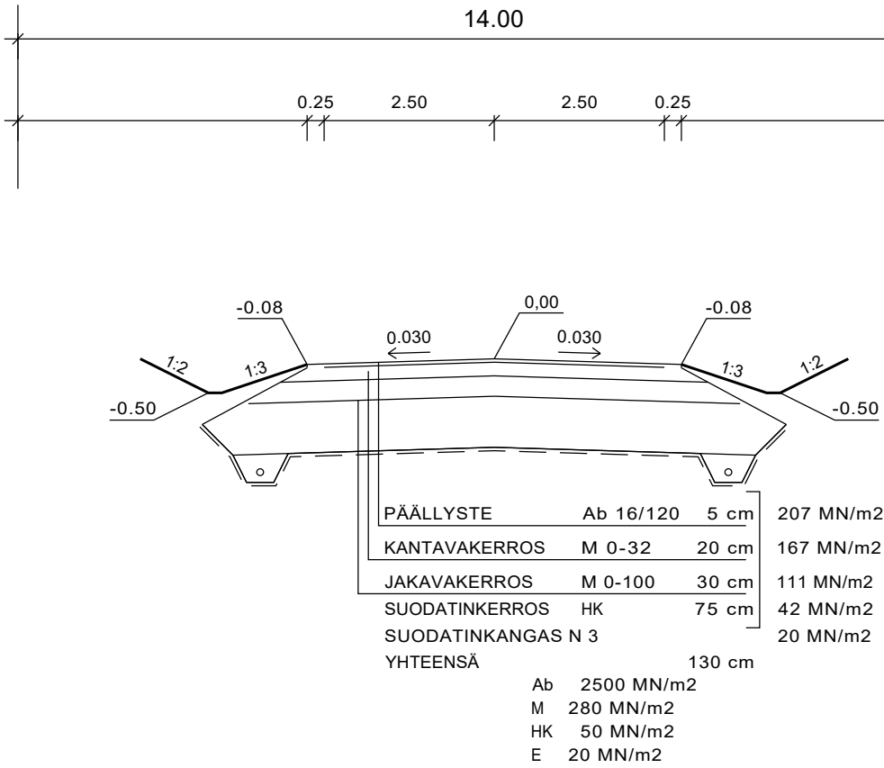
TYYPPIPOIKKILEIKKAUS 1:100
