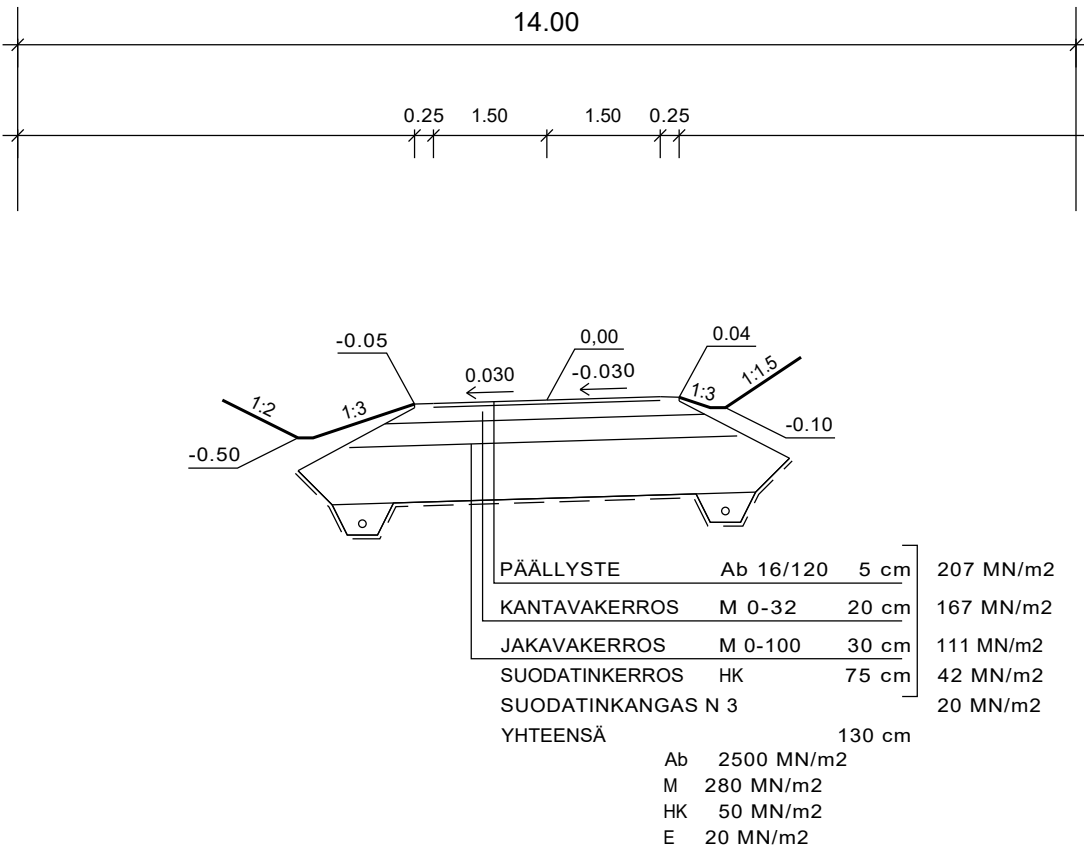
TYYPPIPOIKKILEIKKAUS PAALULTA 120 1:100
